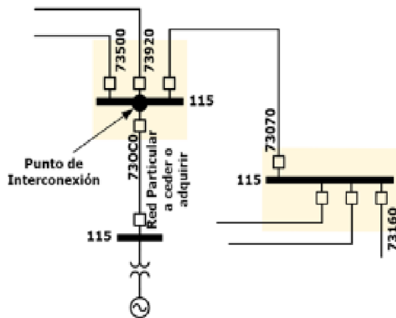
Figura 2 Caso base sin proyecto para P_{RP} .
